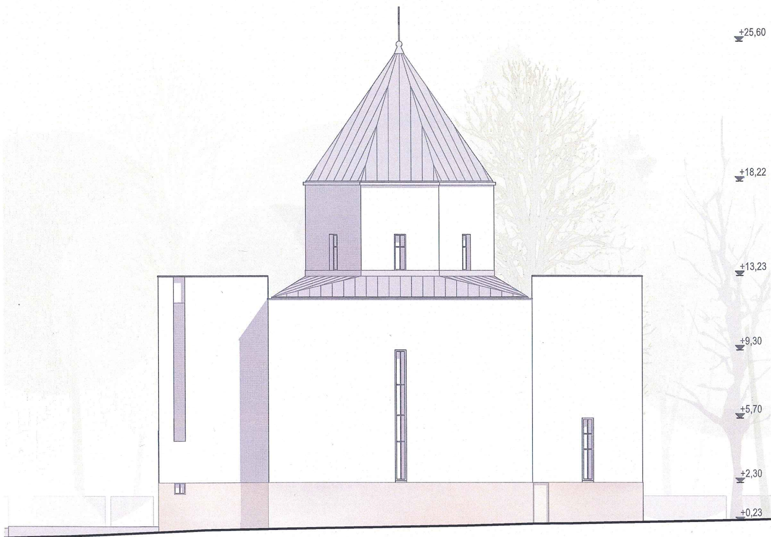
Déli homlokzat
