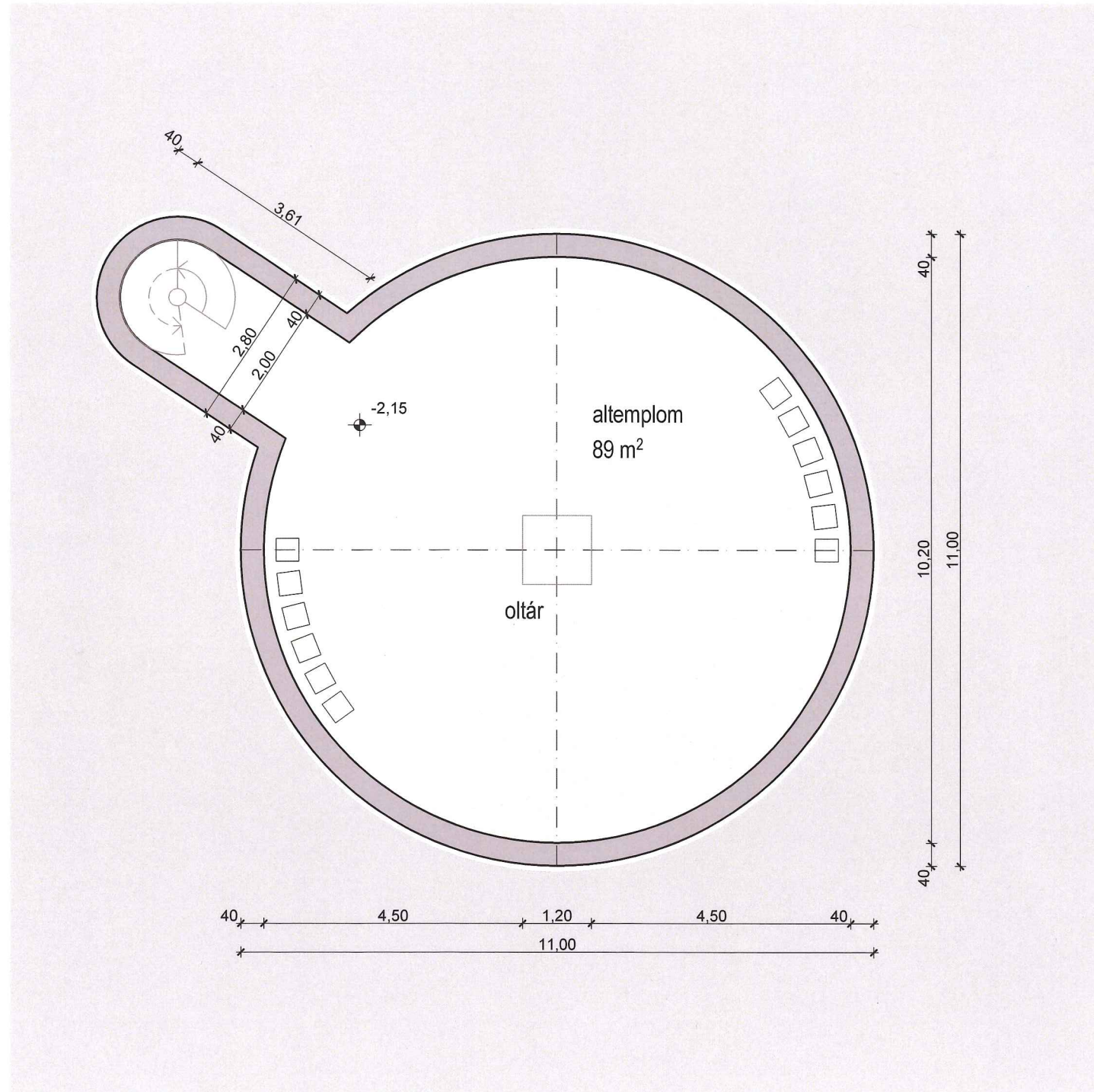
ALPTEPLOM ALAPRAJZ
